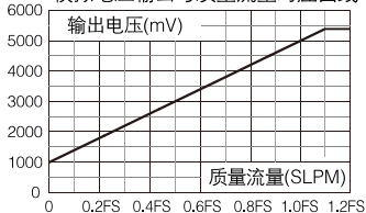
模拟电压输出与质量流量对应曲线
